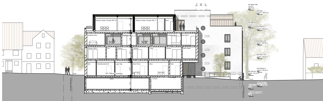
Schnitt B-B
