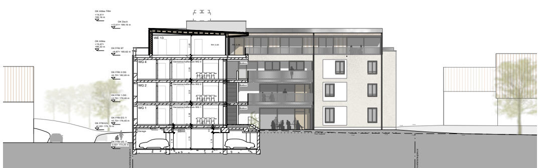
Schnitt C-C
