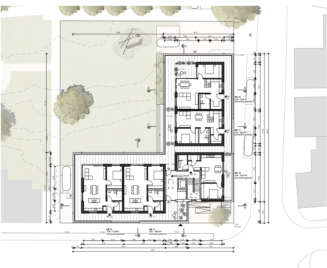
Staffelgeschoss
